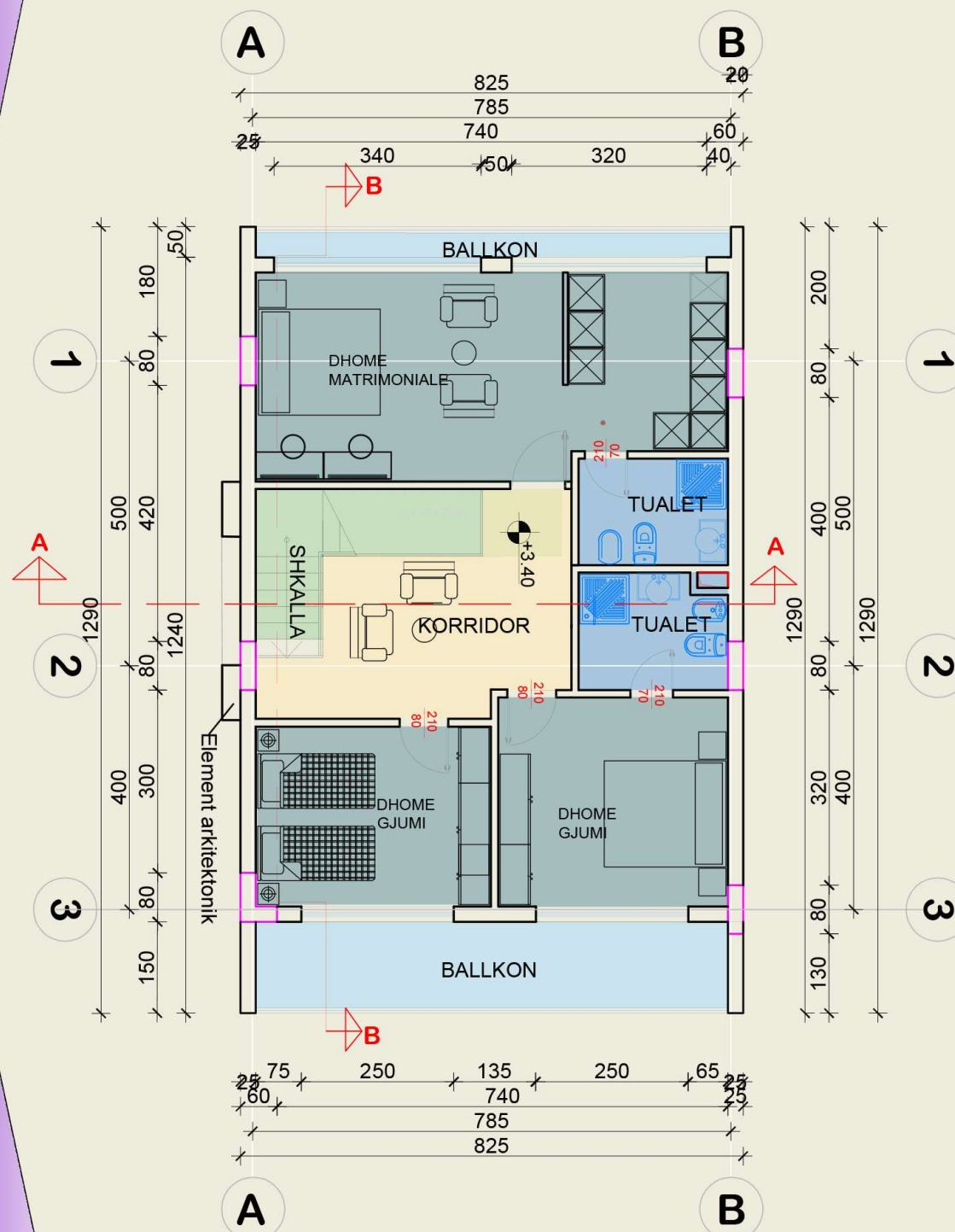
PLANIMETRI KATI 1
