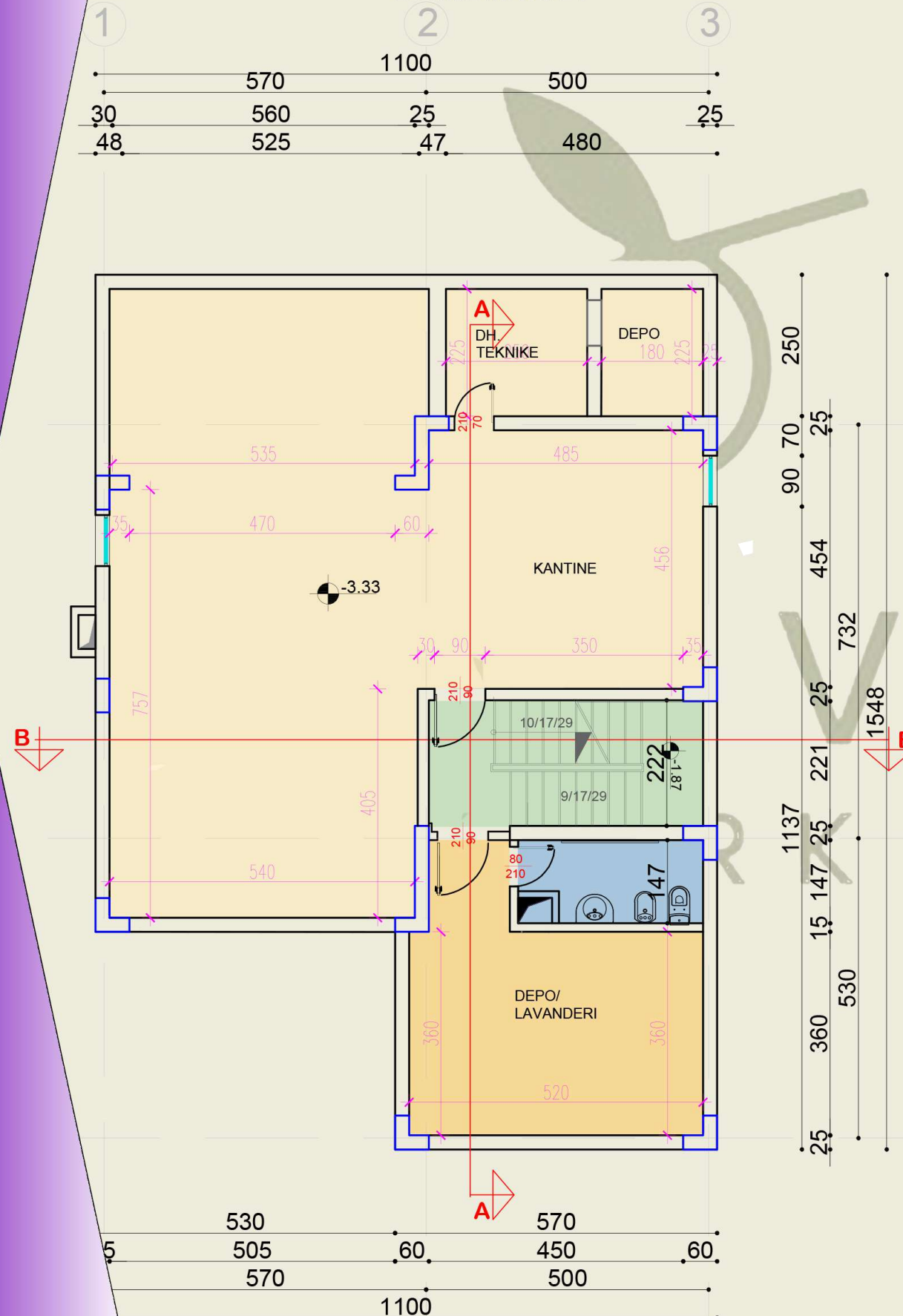
PLANIMETRI KATI -1
