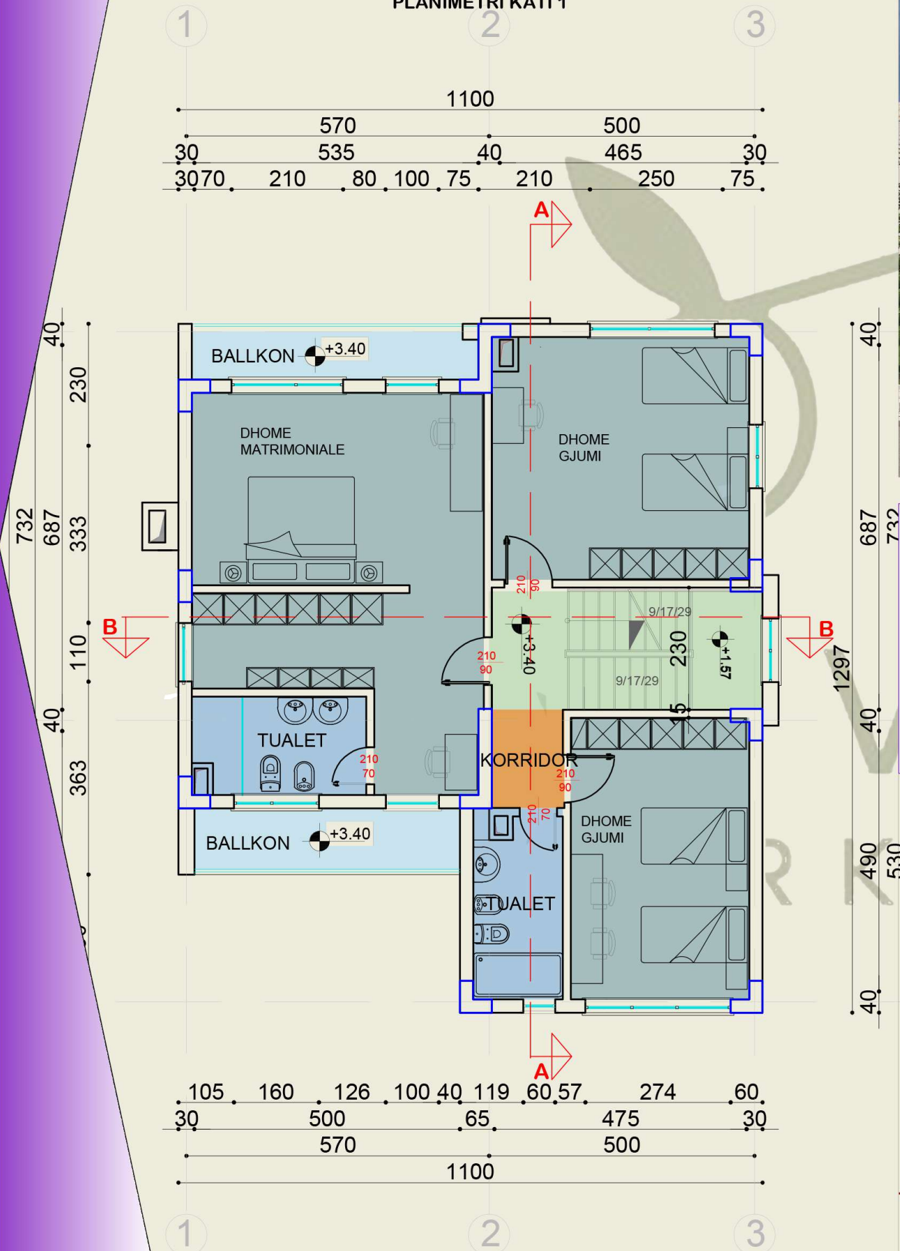
PLANIMETRI KATI 1
